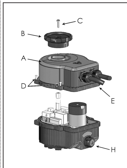
Fig.1 Vista esterna dell'attuatore
